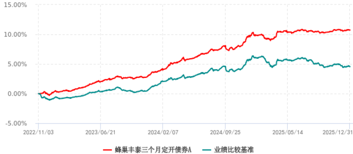
蜂巢丰泰三个月定开债券A累计净值增长率与业绩比较基准收益率历史走势对比图 (2022年11月03日-2025年12月31日)
