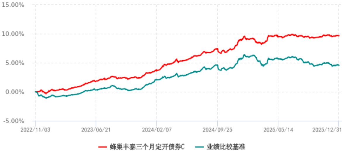
蜂巢丰泰三个月定开债券C累计净值增长率与业绩比较基准收益率历史走势对比图 (2022年11月03日-2025年12月31日)
