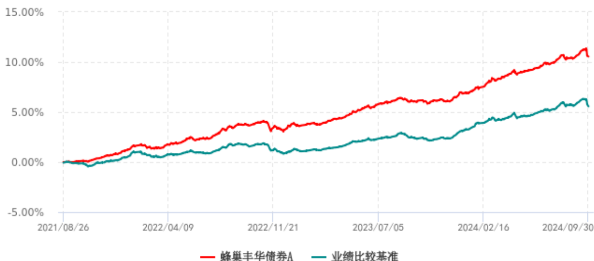
蜂巢丰华债券A累计净值增长率与业绩比较基准收益率历史走势对比图 (2021年08月26日-2024年09月30日)
